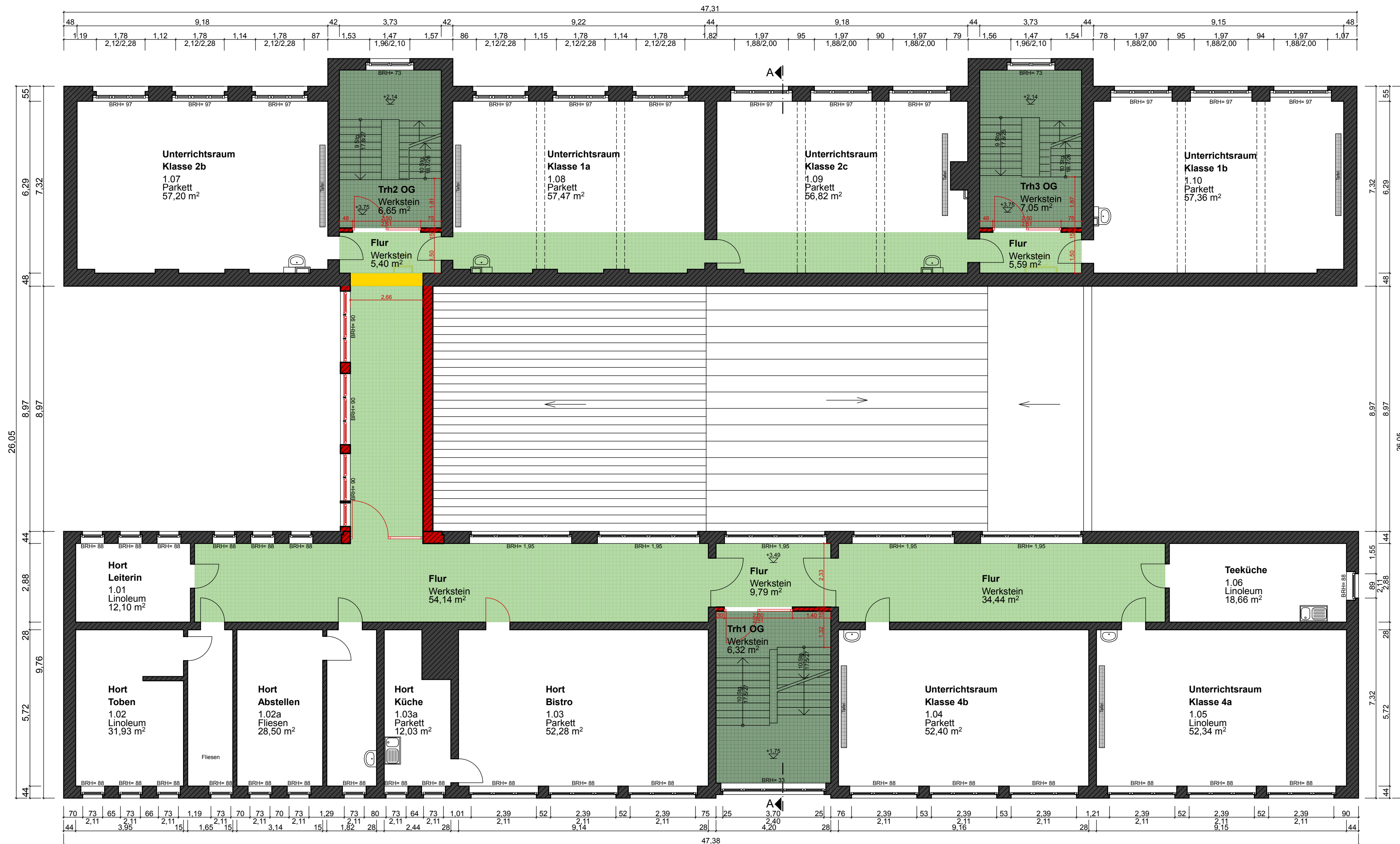
Grundriß Obergeschoß
