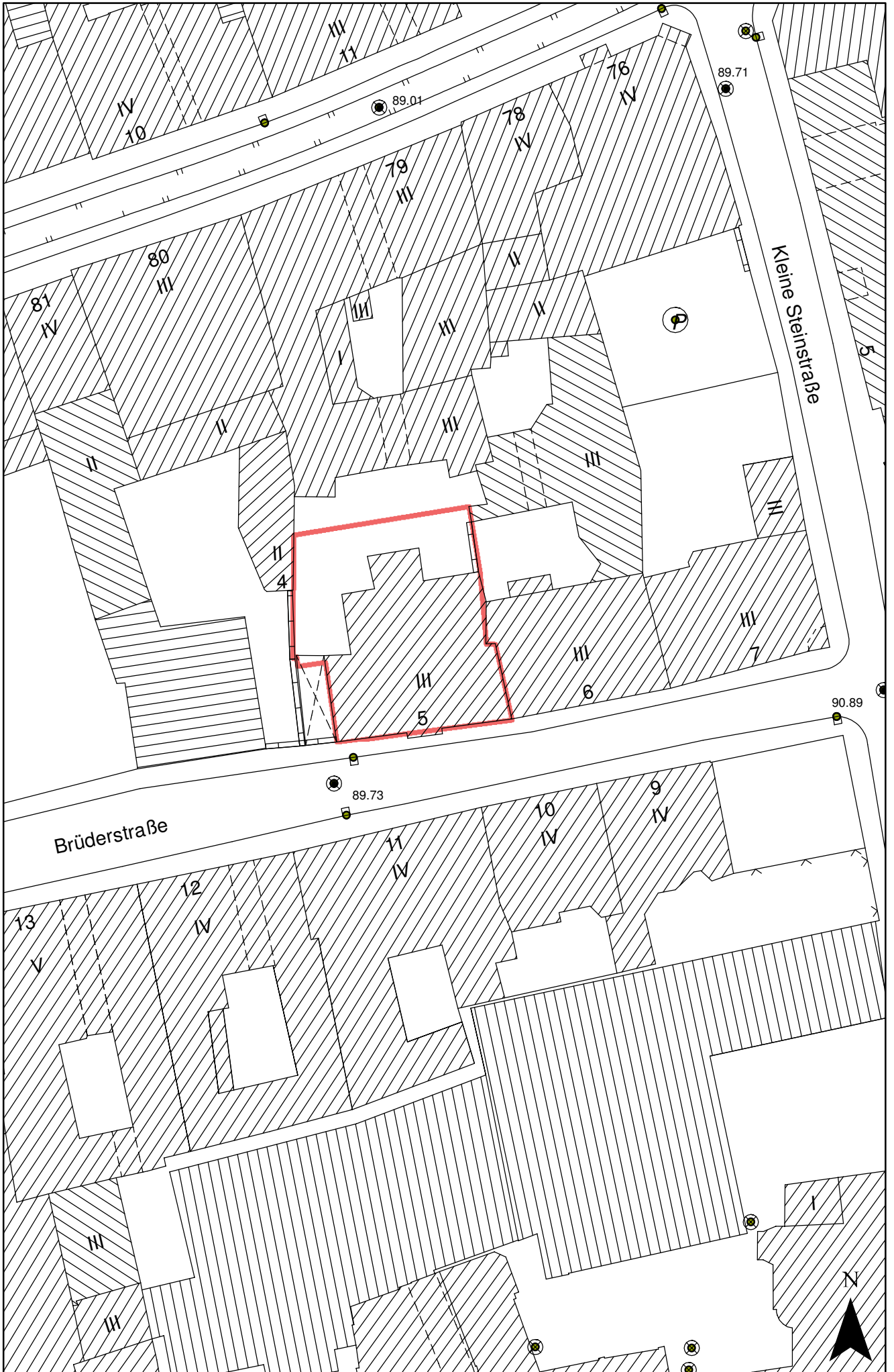
Lageplan M 1:500
