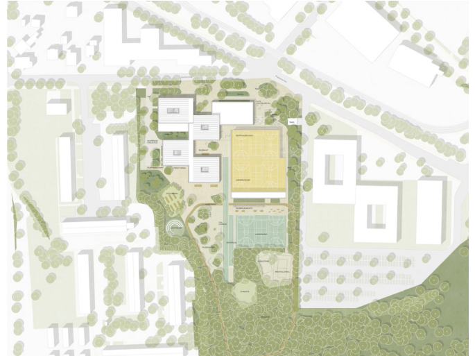
„Gymnasium Pappelallee Potsdam“ Objektplanung Freianlagen, derzeit LPH3+4 Hochbau: ASW Atelier Schmelzer Weber
